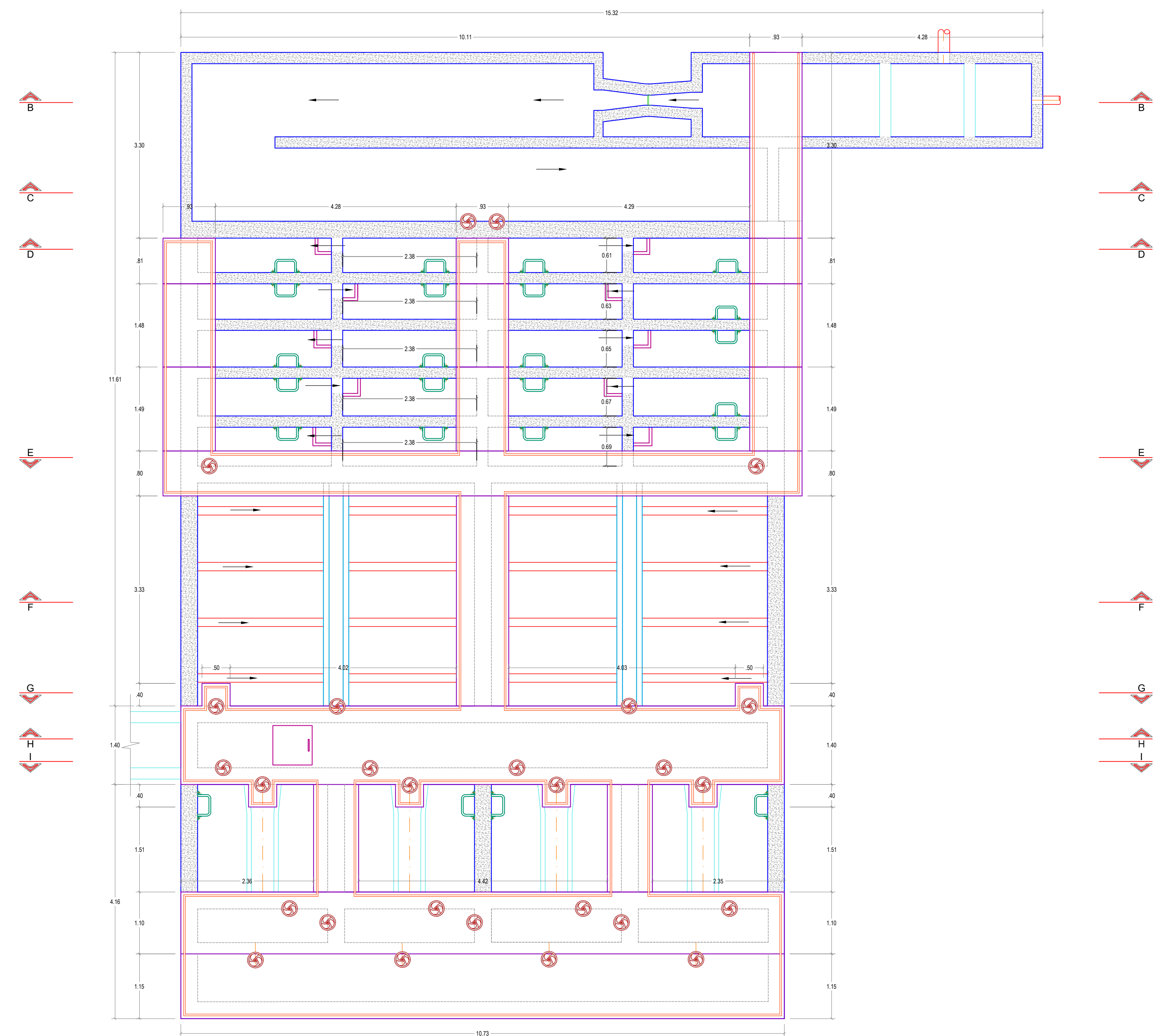
VISTA EN PLANTA NIVEL DE PASARELAS ESC 1 : 50
