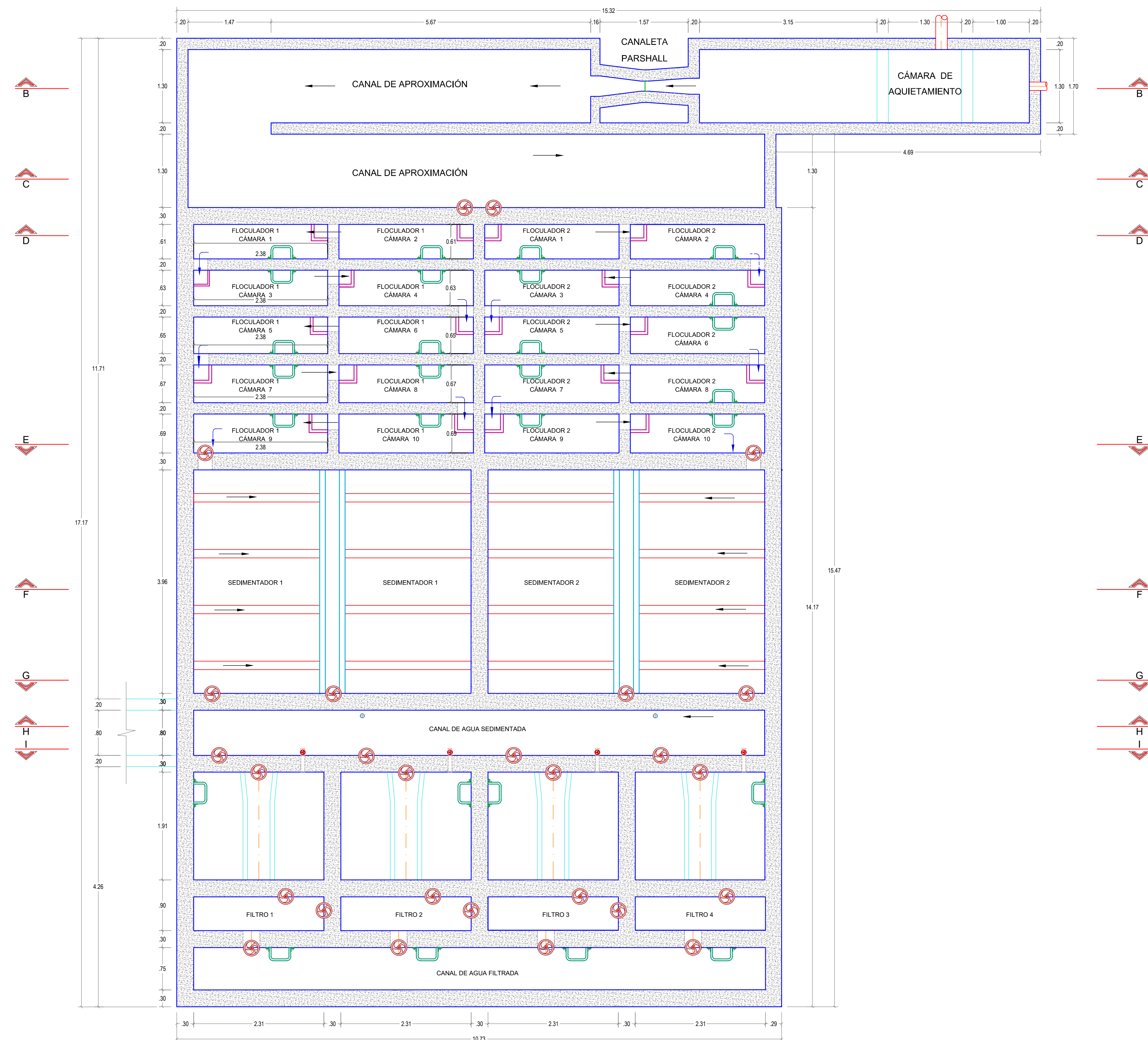
VISTA EN PLANTA DEBAJO DE PASARELAS ESC 1 : 50
