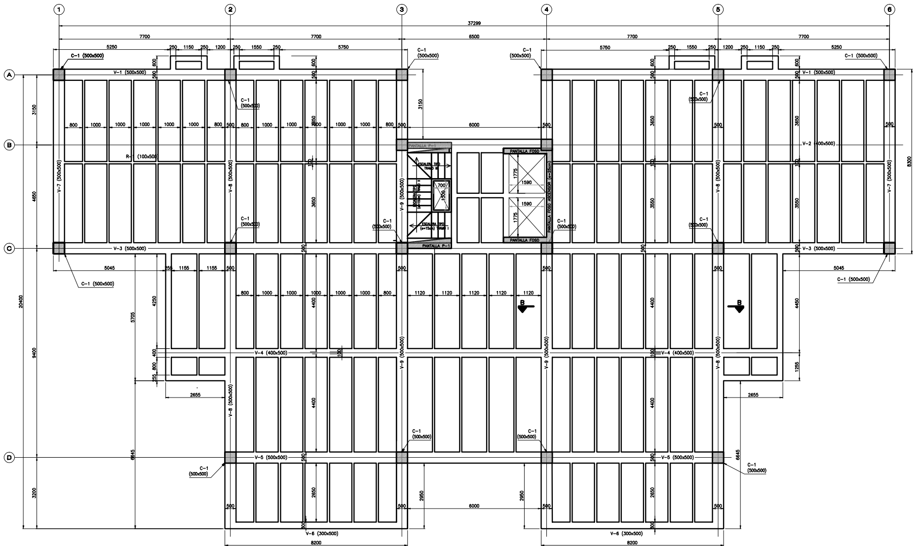
PLANTA ENTREPISO TRADICIONAL- ALIGERADO DIMENSIONES ESC.:1:75
